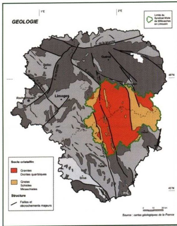
Roche métamorphique.
