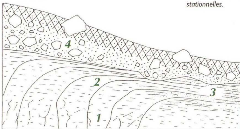
Arènes sur roche cristalline - coupe schématique. D'après B. Valadas (1987)
